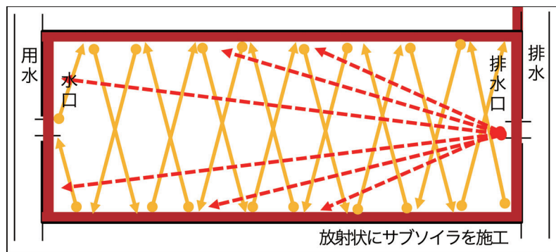
図1 放射状+短辺対角線状の暗渠施工
