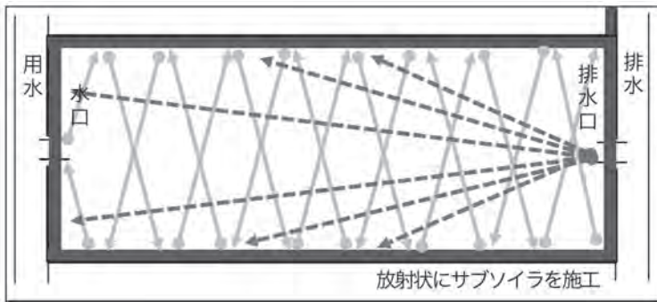
図1 放射状+短辺対角線状の暗渠施工
