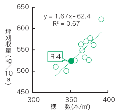
図2 穂数と収量
